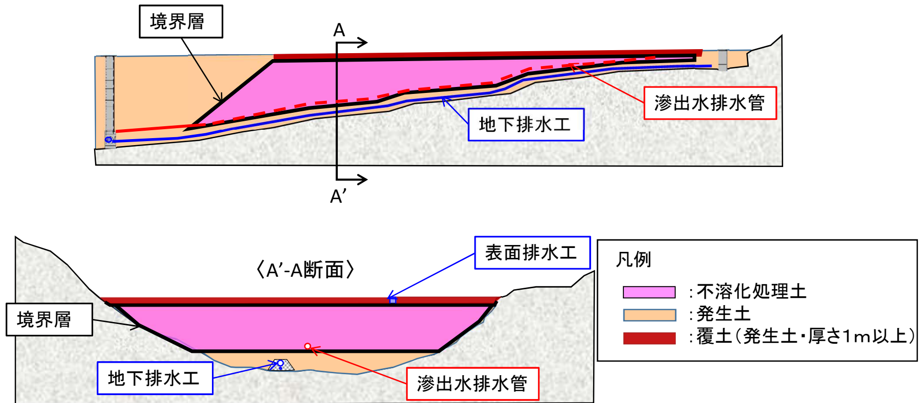
【活用箇所縦断図】
