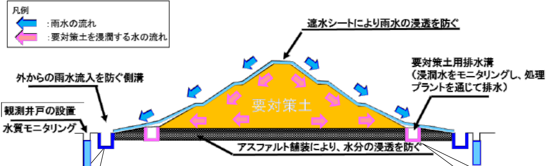
図：要対策土仮置き場における盛土計画
