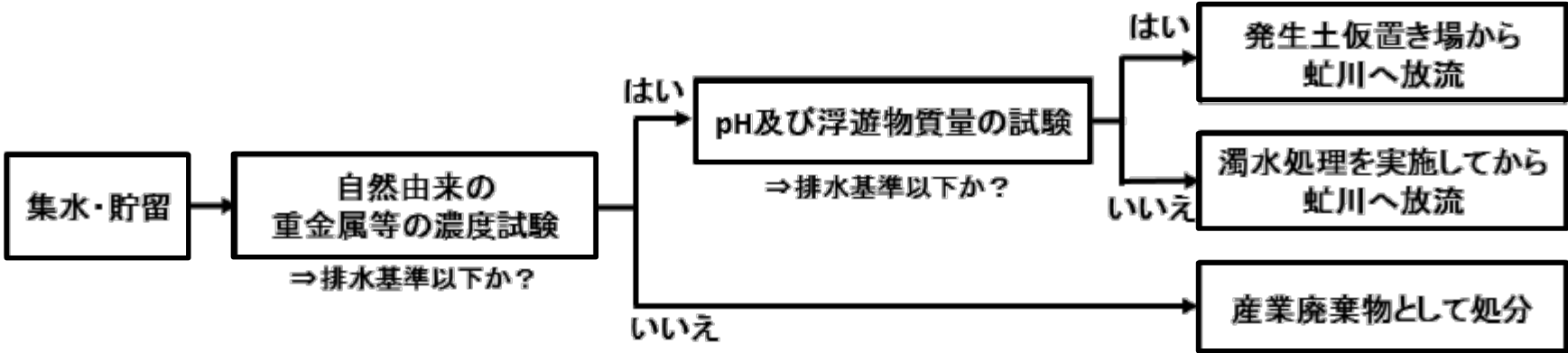
図：排水処理のフロー
